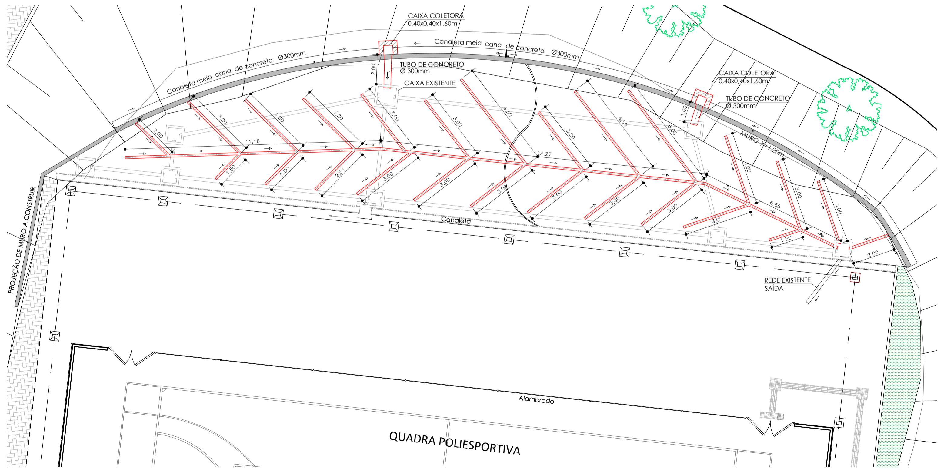
PLANTA BAIXA ESC.: 1/100
